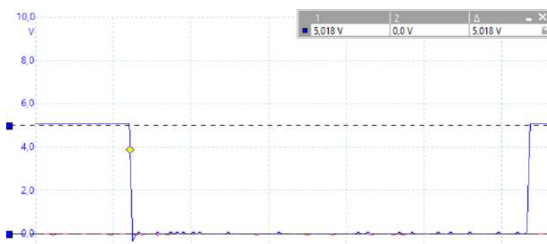
Figure -24- visualisation de signal d'interruption sur le picoscope.
