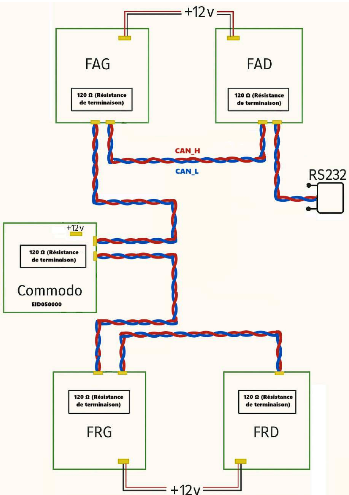
Figure -21- Architecture du réseau CAN du module CAN01A avec les résistances de terminaison et alimentation 12V.
