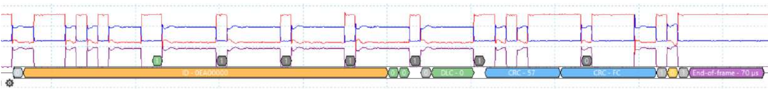
Figure -33- Trame de retour depuis le MCP25050
